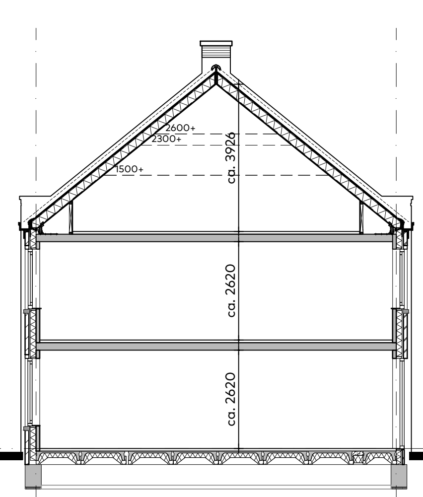
principe doorsnede tussen
