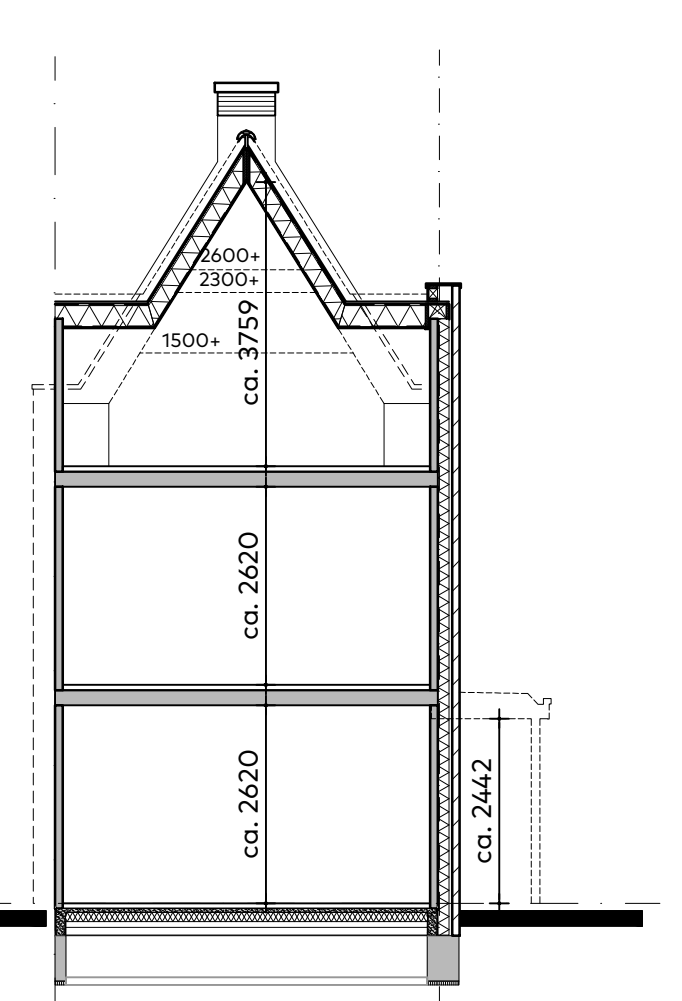
principe doorsnede tuitgevel
